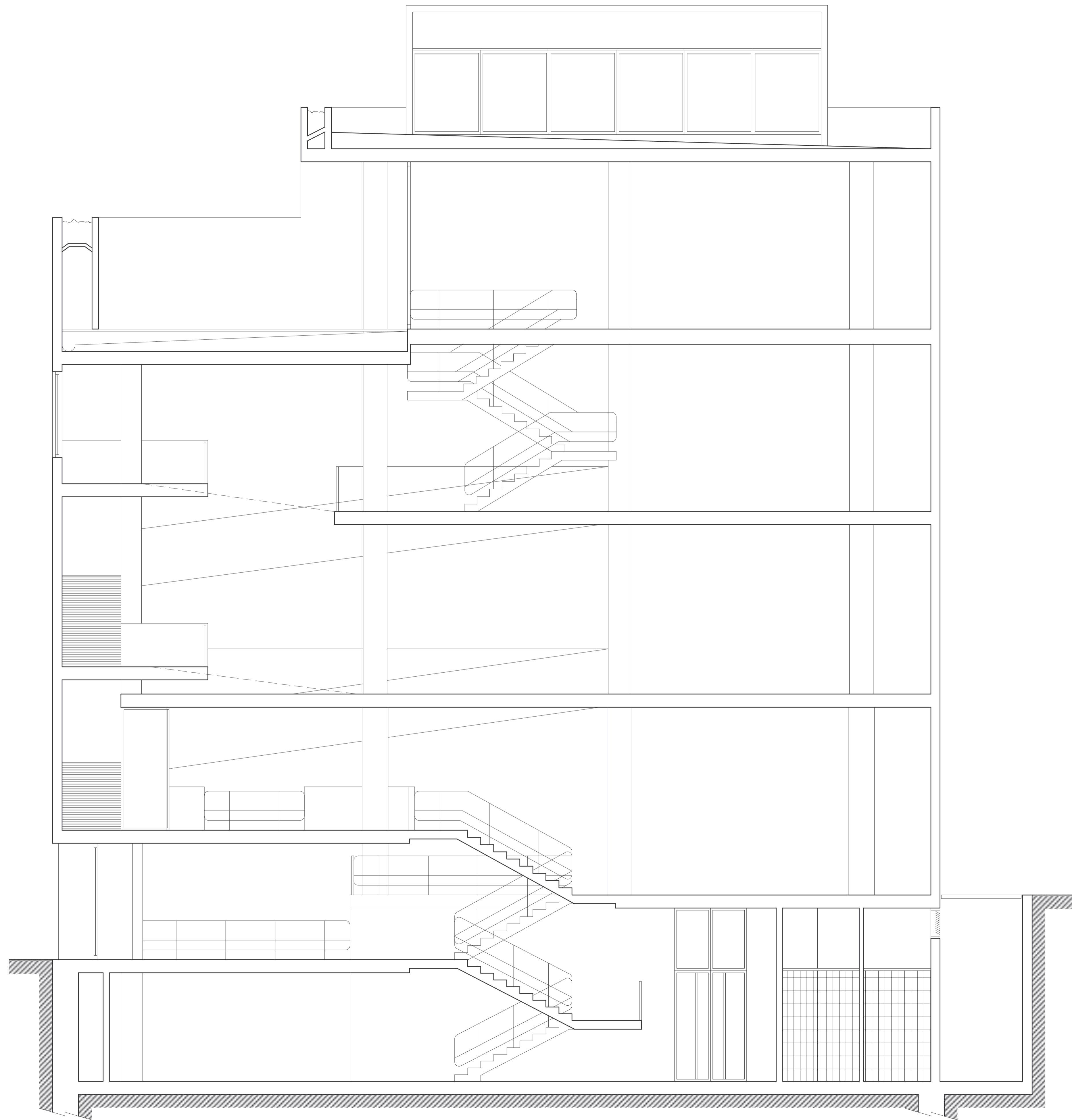
SECCIO A-A
